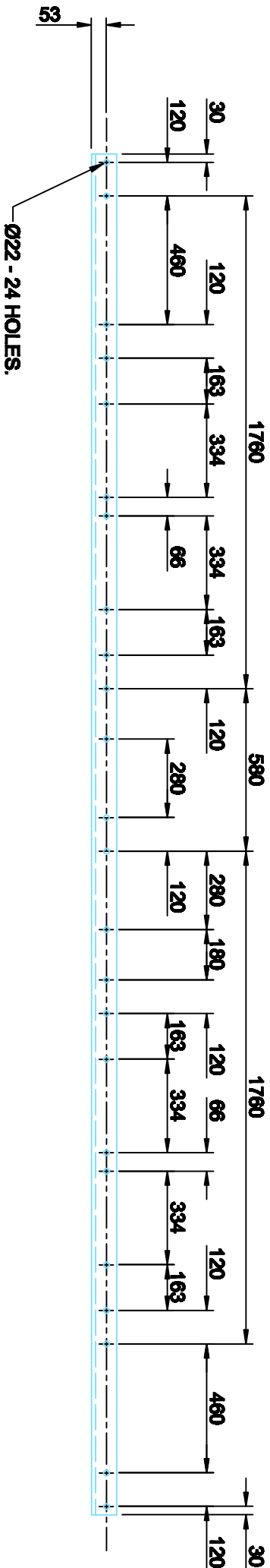
ITEM 6. 4860 LONG x 150 x 90 x 15 UNEQUAL ANGLE.
